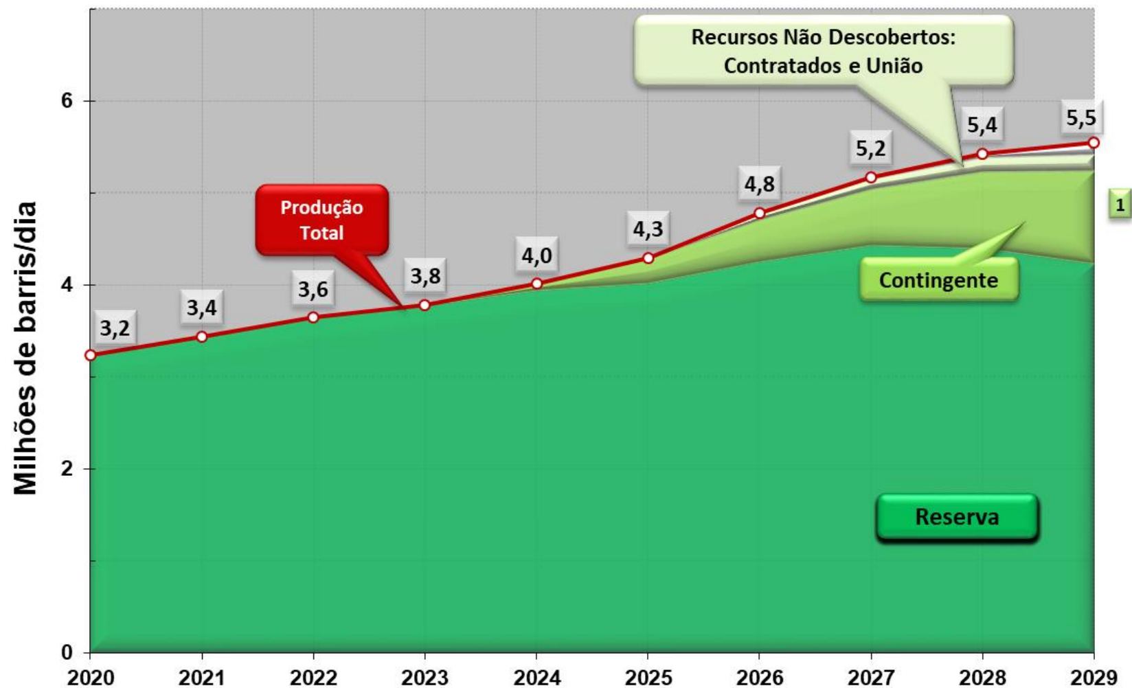
Gráfico 5-1. - Previsão de produção diária de petróleo nacional
